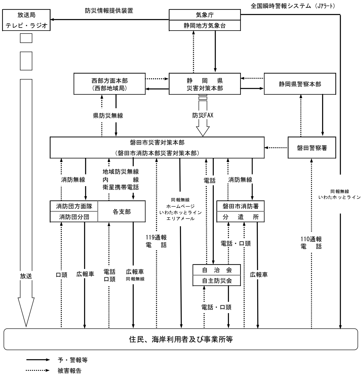
図 6-1 情報受信・伝達系統図
