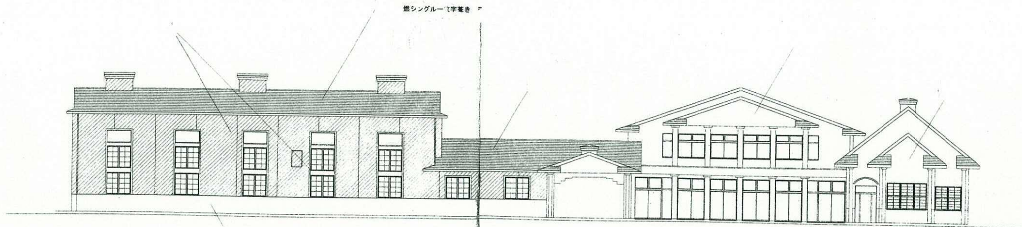
東面 立面図 A2=1/200
