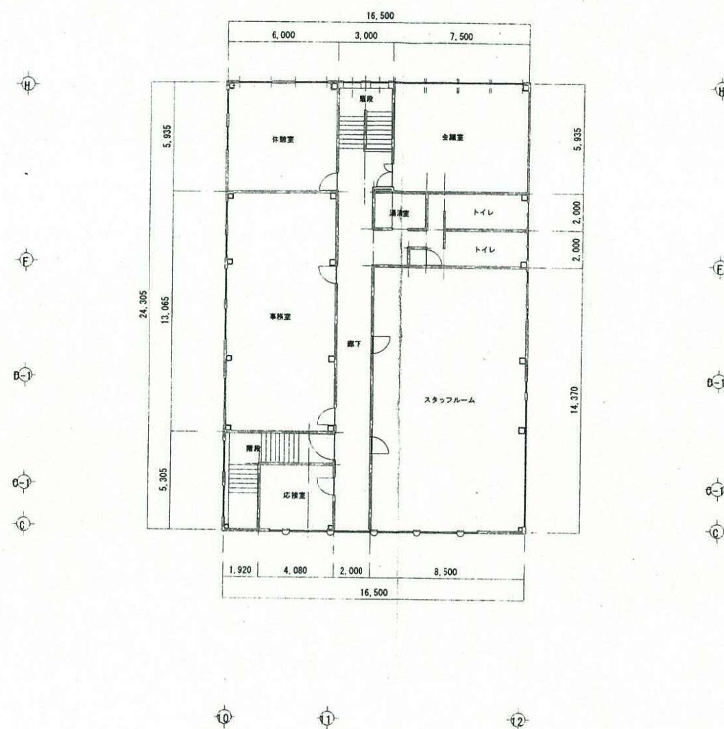
現況 2階平面図 A2=1/200
