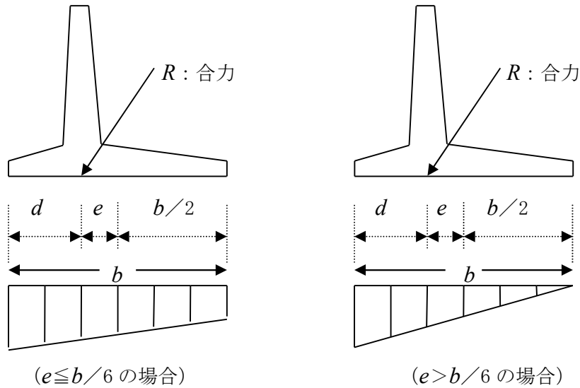
擁壁底面の地盤反力
