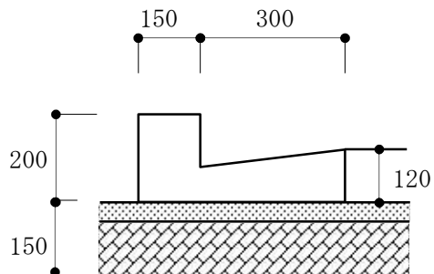
L 型側溝
