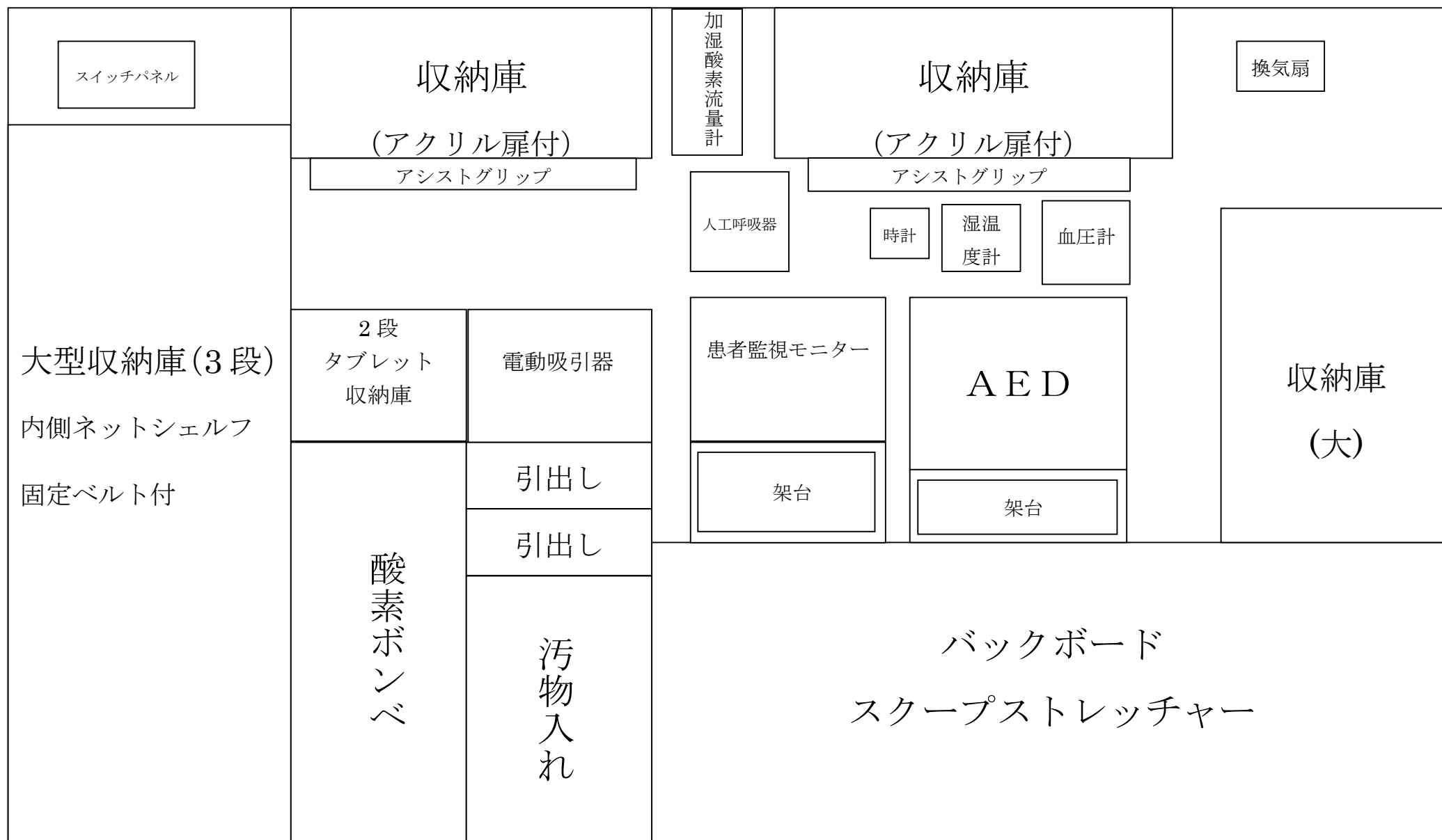
患者室右側（運転席側） 救急資器材積載概要図
