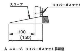
A スロープ、ワイパーガasket 詳細図
