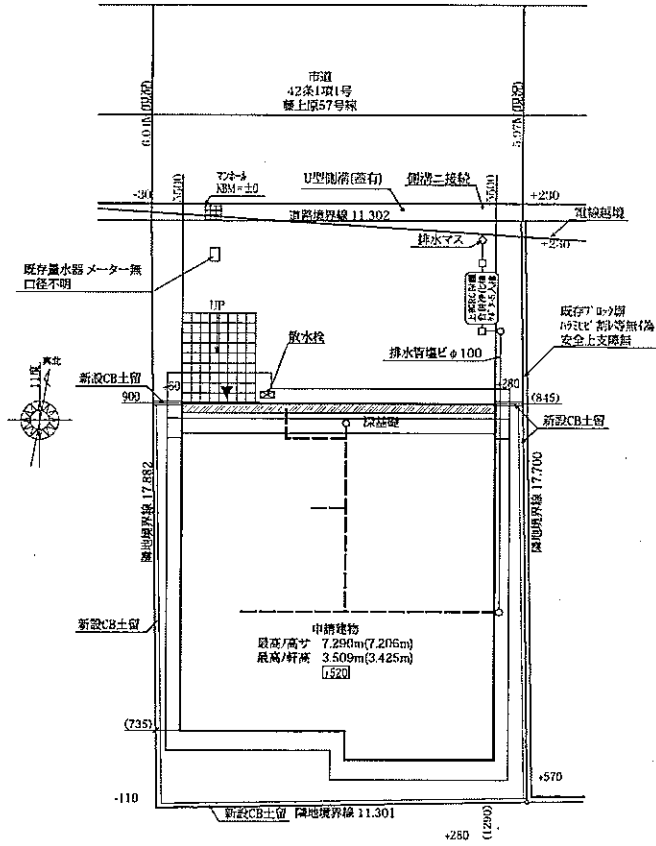
平面図
