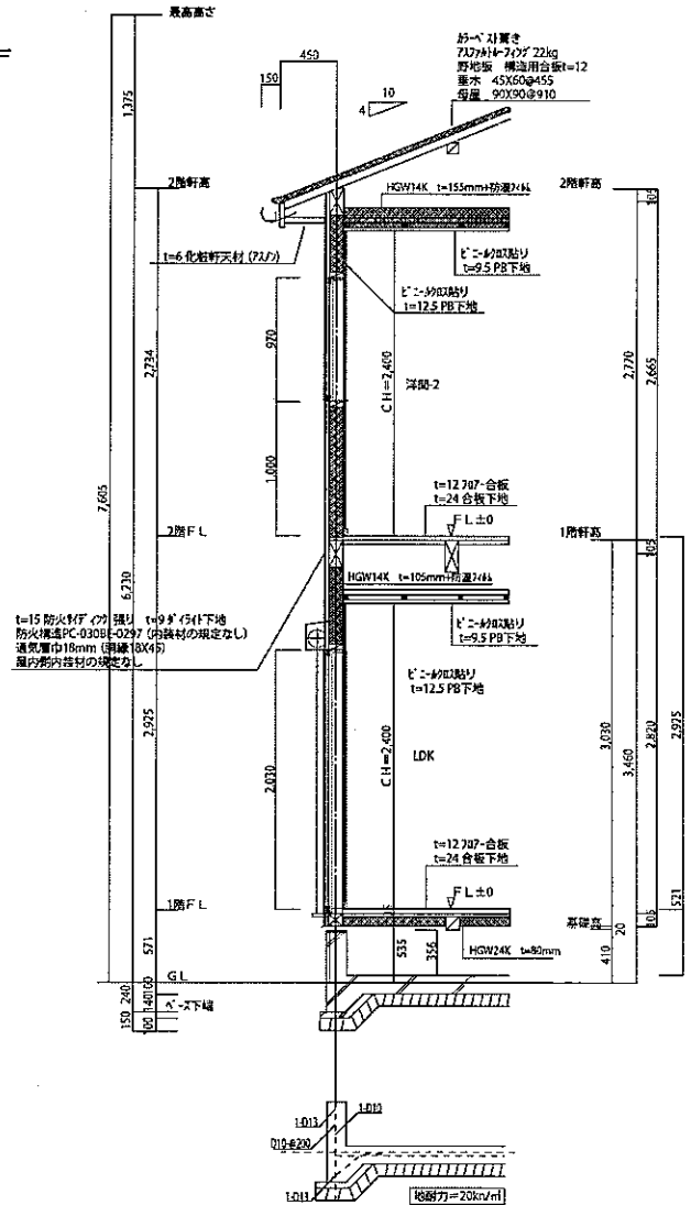
断面図
