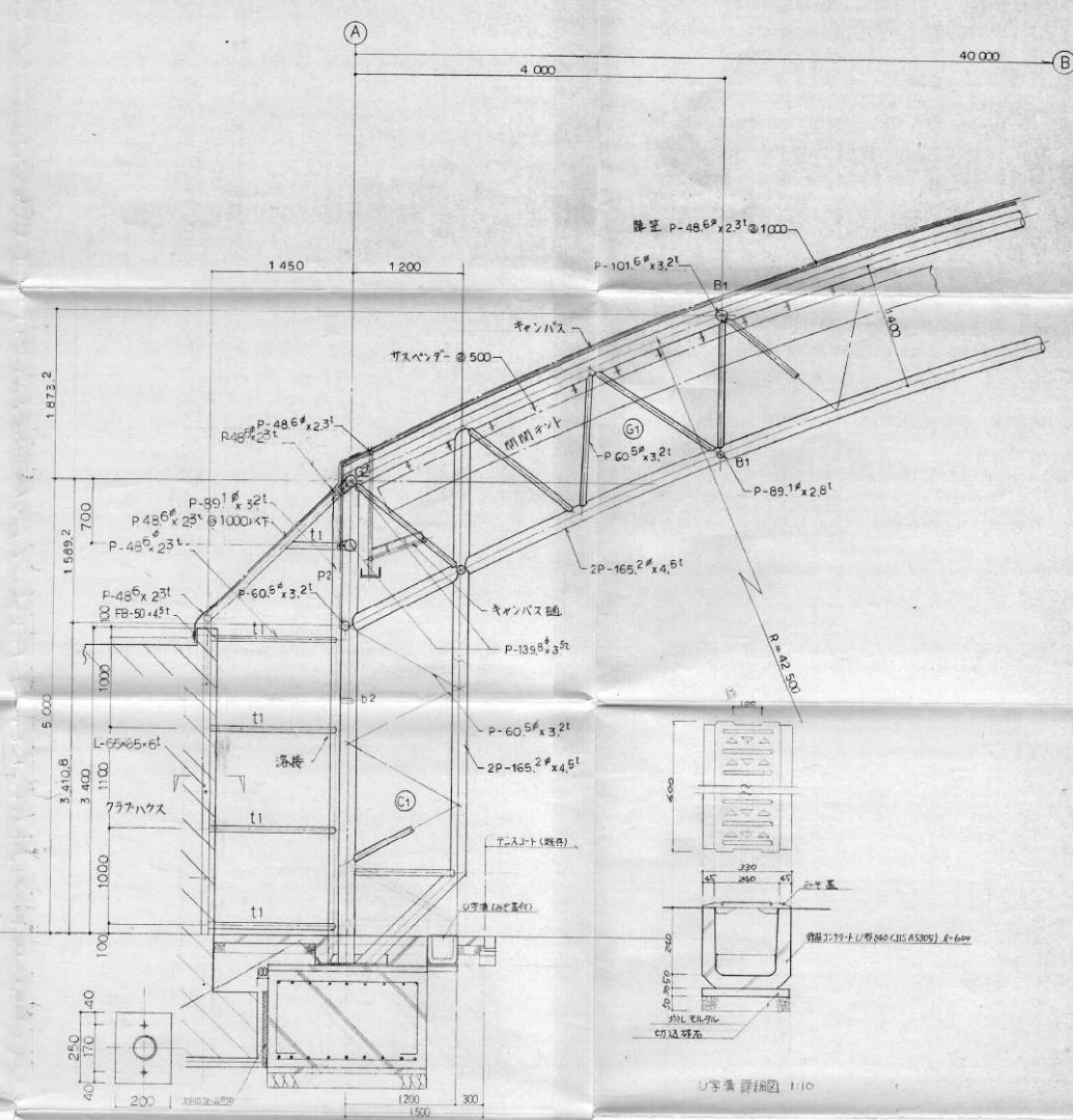
BASE 詳図 (1/10)
