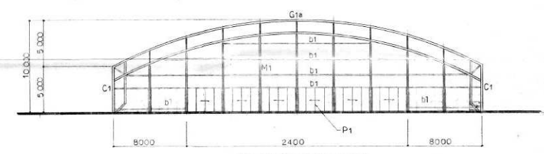
側立面図 S-1:200
