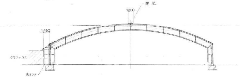
断面図 S-1:200
