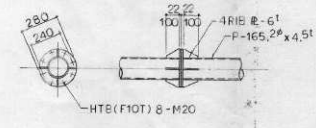
JOINT 詳細図 S=1:20
