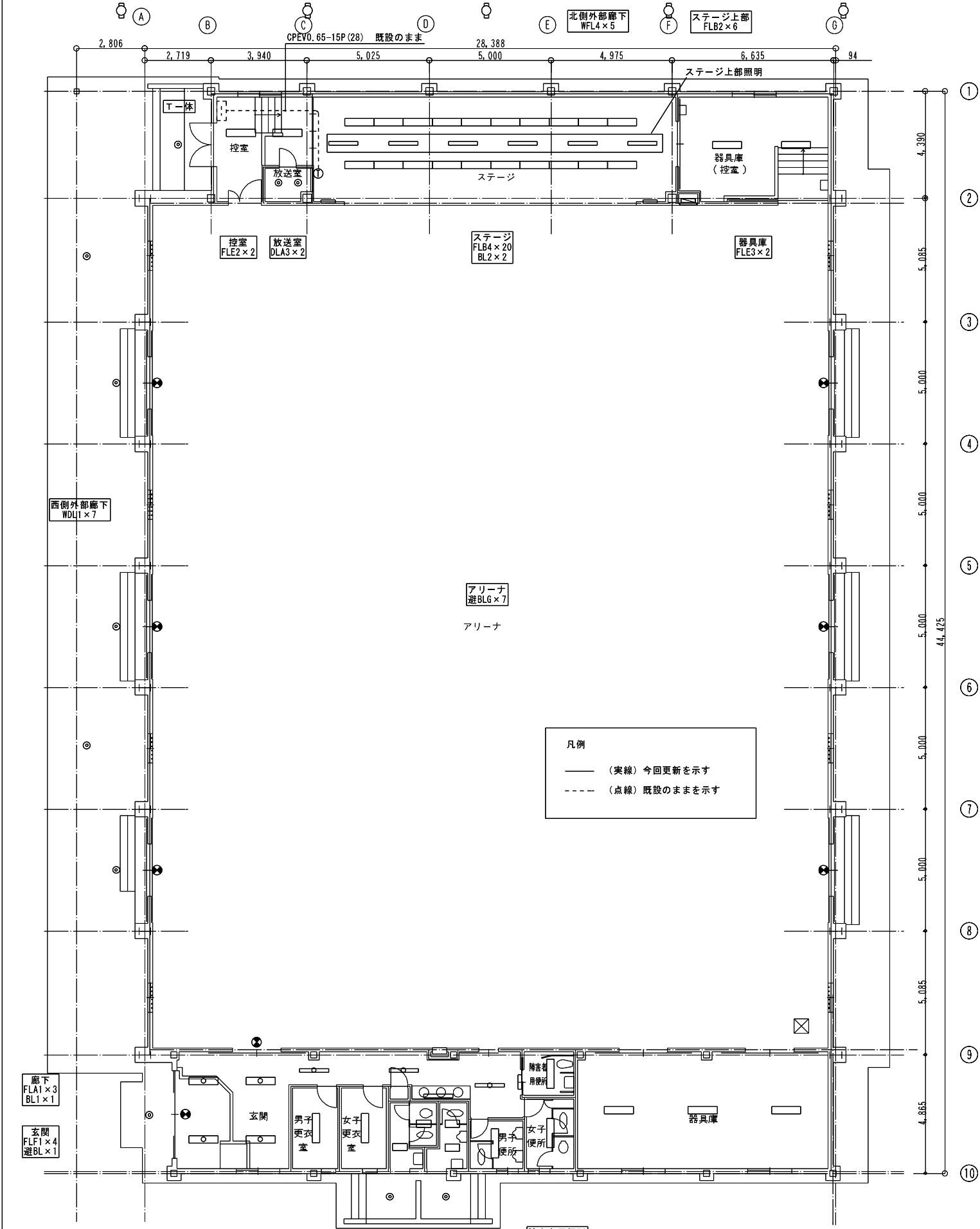
屋内運動場 1階平面図 (改修後)
