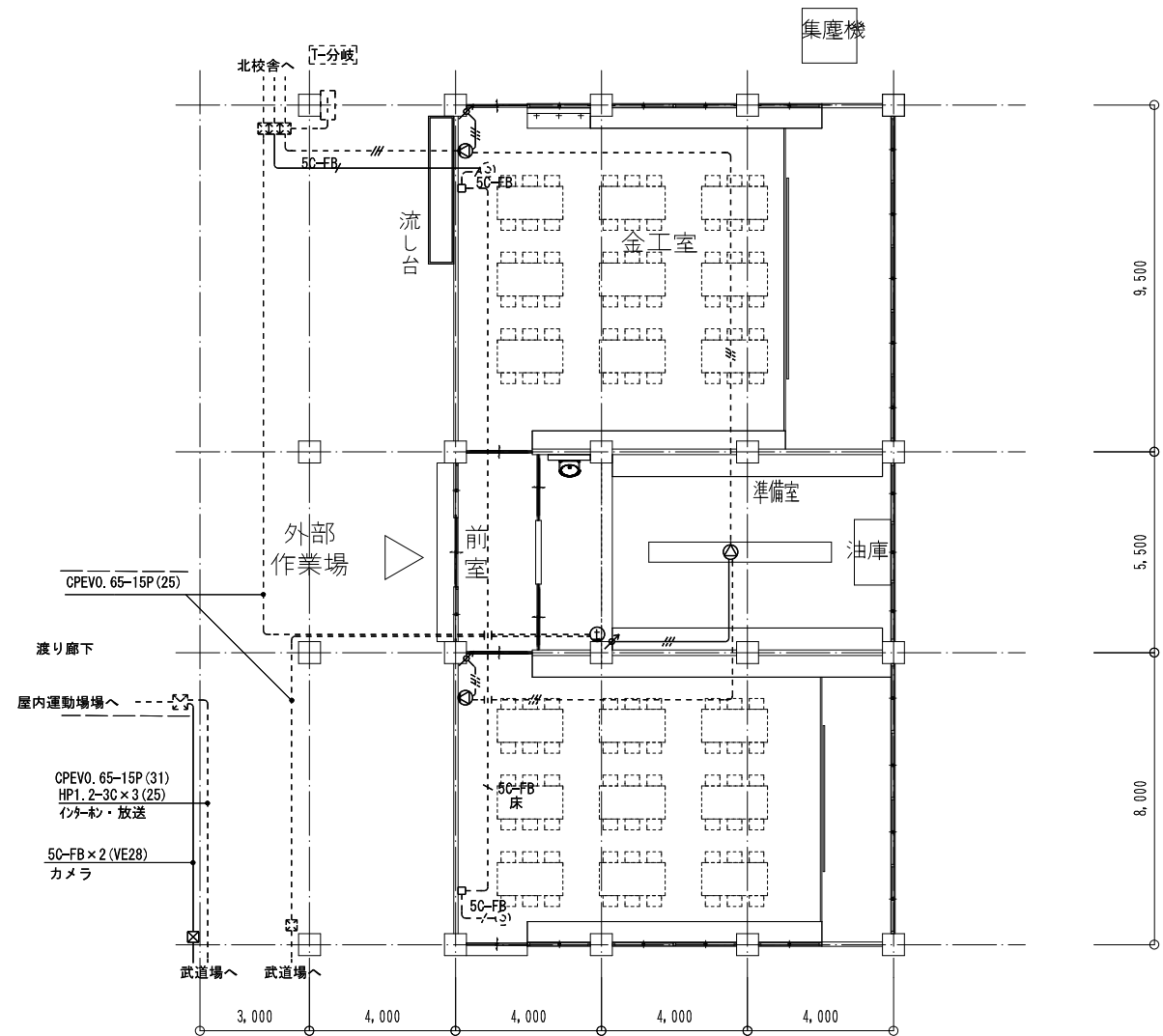
( 現況 ) アトリエ棟平面図
