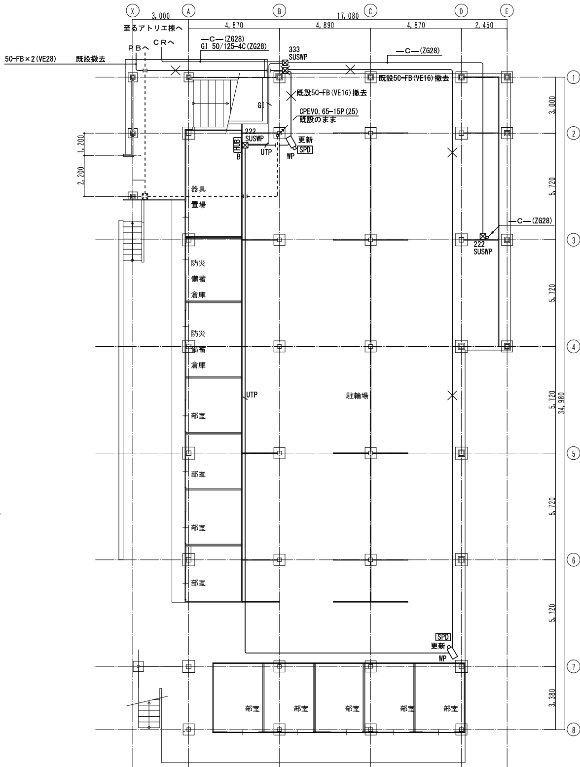
武道場 1 階平面図
