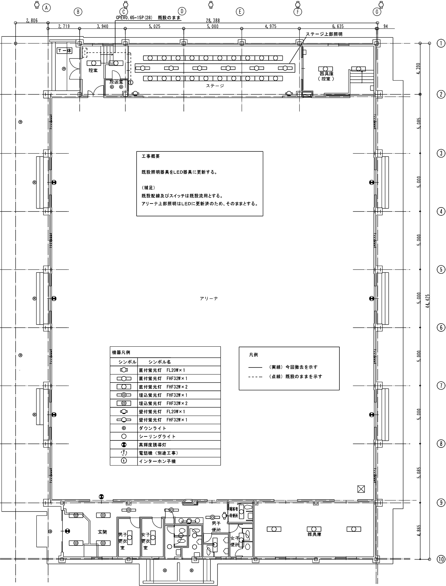
屋内運動場 1階平面図 (現況)
