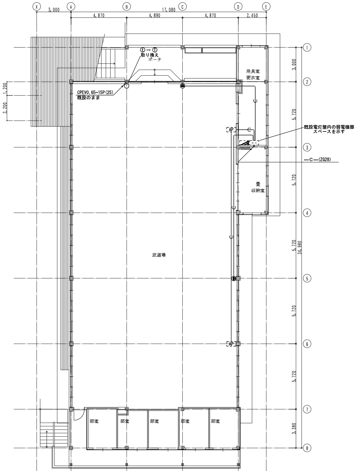
武道場 2 階平面図
