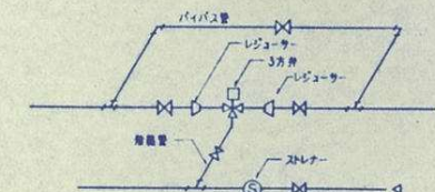
3方弁装置 組立て要領
