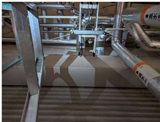
既設減算メーター 50 A 検満期限：令和 9 年 1 月
