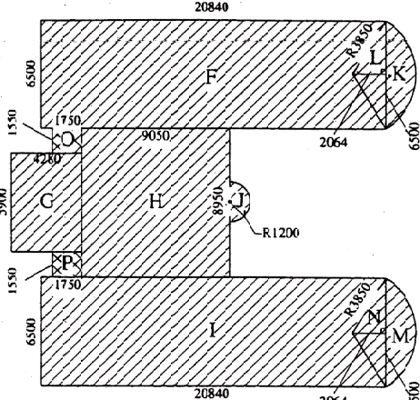
2階求積図
