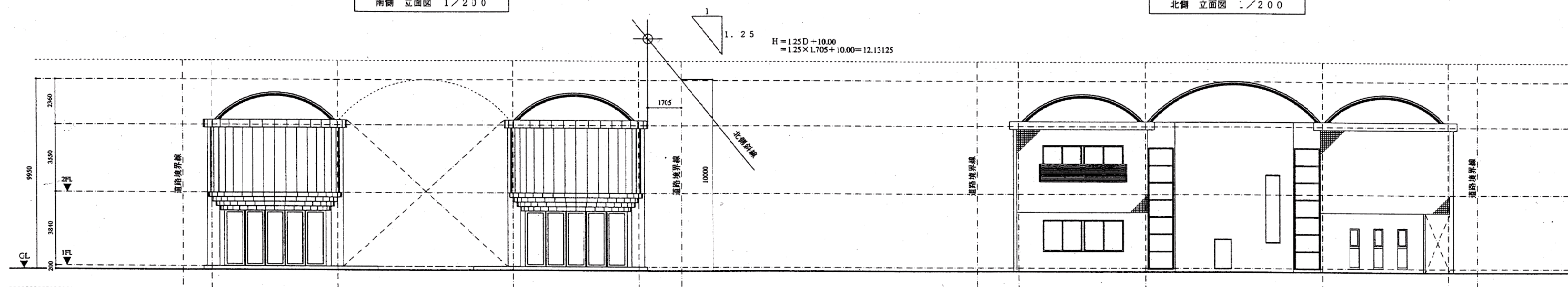
東側 立面図 1/200
