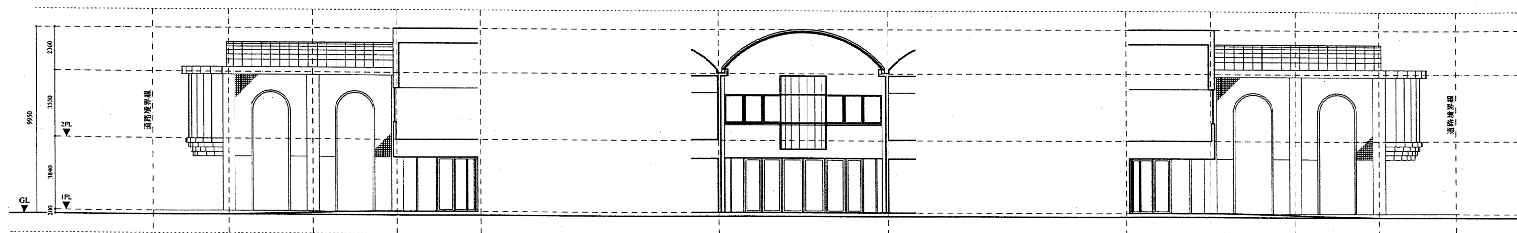
中庭部分南側 立面図 1/200
