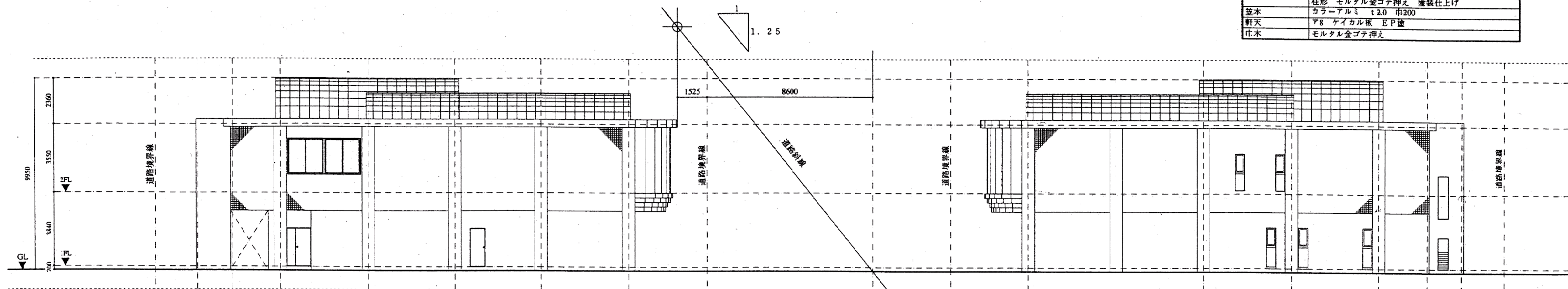
南側 立面図 1/200
