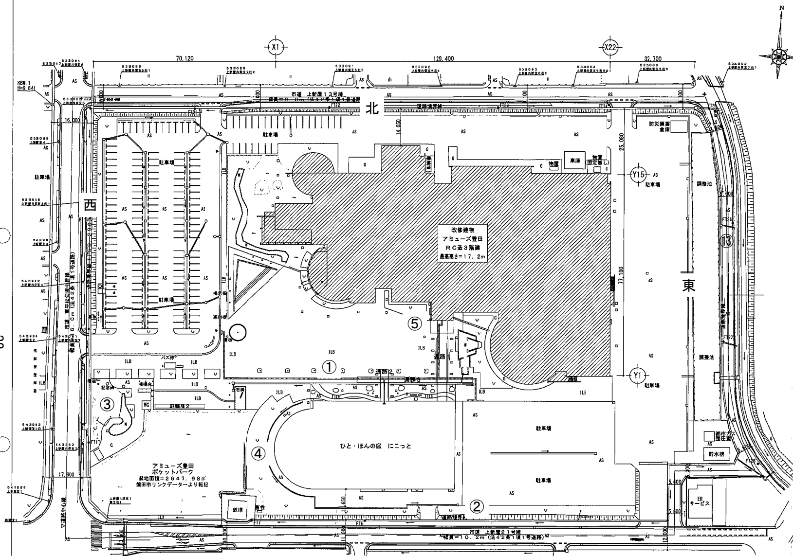
配置図 S=1/1000
