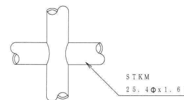
接合部詳細 S = 1 / 3
