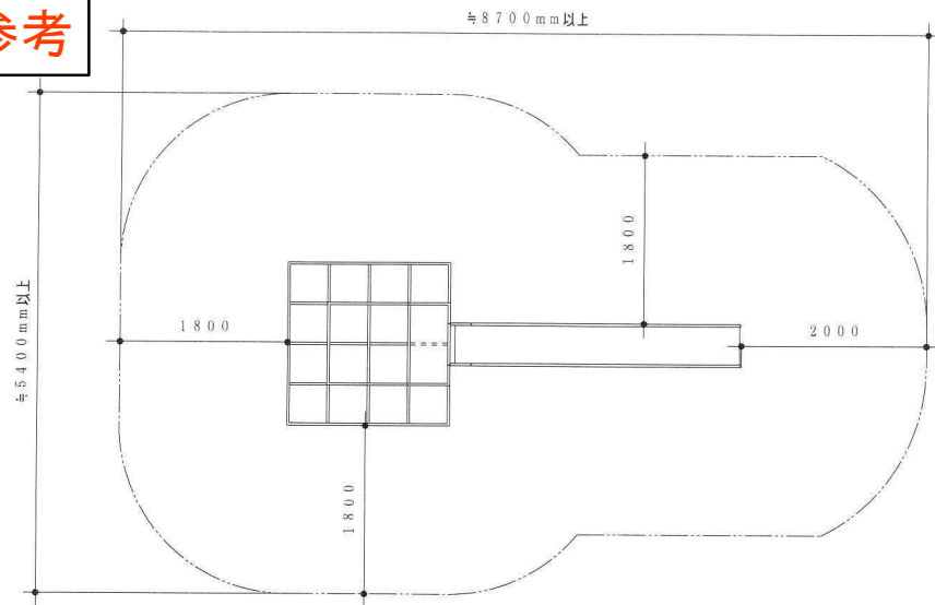
安全領域図 S = 1 / 6 0
