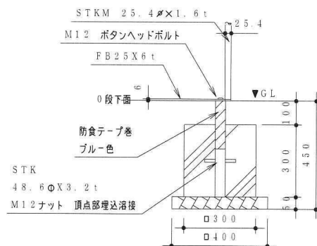
ジャングル部基礎図 S = 1 / 1 5
