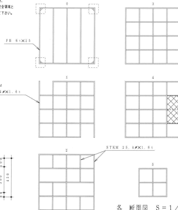
各断面図 S = 1 / 4 0
